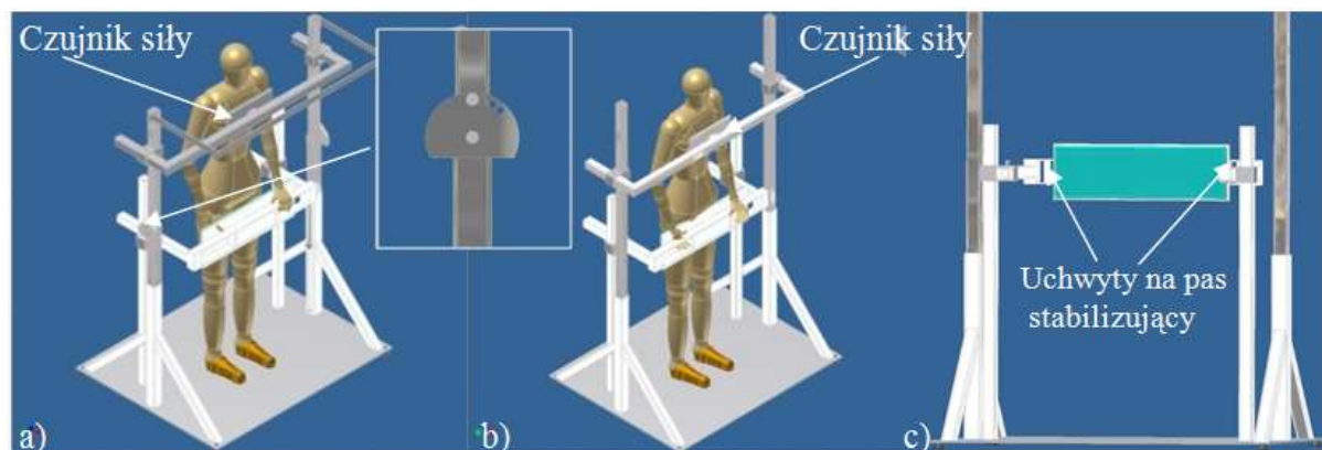
Rys. 4. Koncepcje urządzeń a) koncepcja trzecia, b) koncepcja czwarta, c) rama stabilizacyjna
