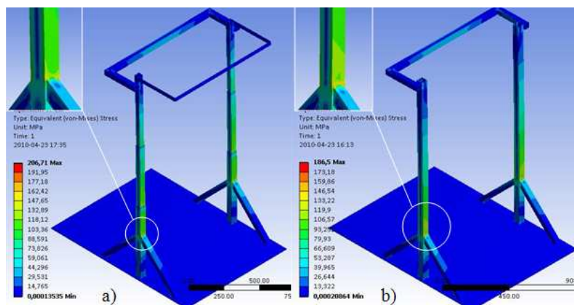
Rys.7. Mapa naprężeń zredukowanych według hipotezy Hubera-von Misesa dla I wariantu obliczeń: a) koncepcja trzecia, b) koncepcja czwarta
