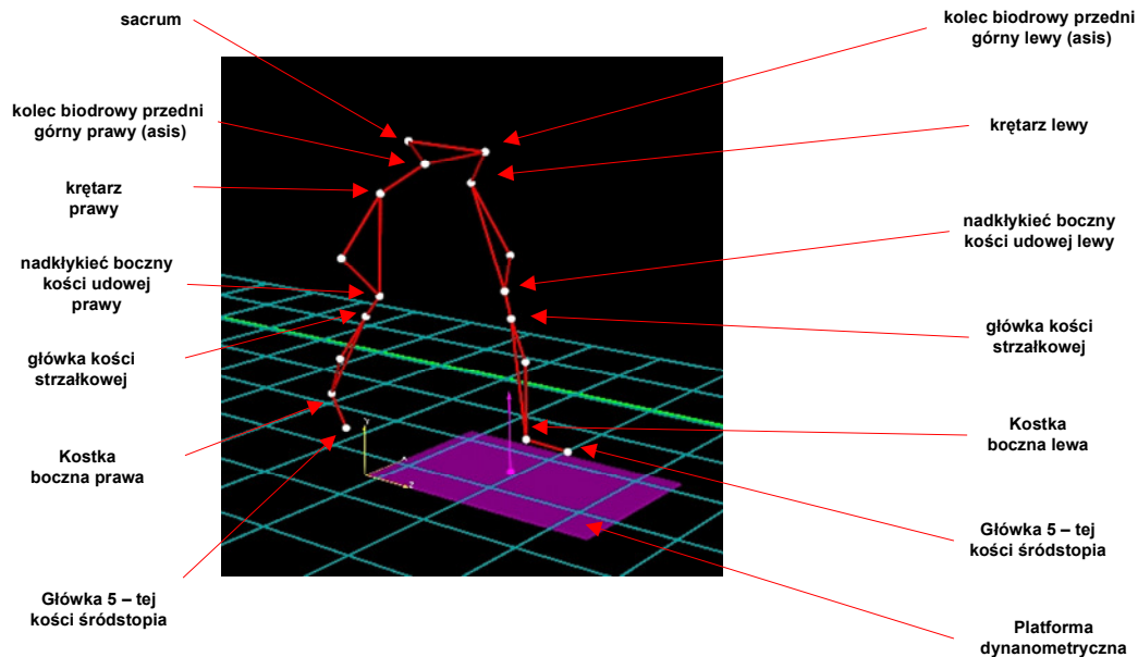
Rys. 4. Schemat modelu 3D a pakiecie SMART Tracker.
