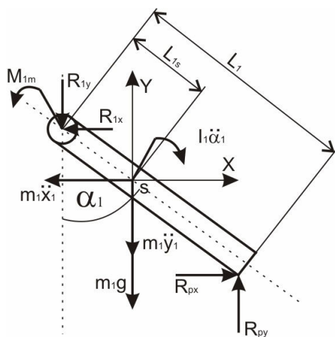
Rys. 3. Rozkład sił działających na stopę
